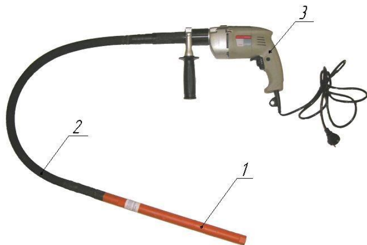
Рисунок 1. Вибраторы электрические глубинные ручные портативные ВИ-120, ВИ-121
