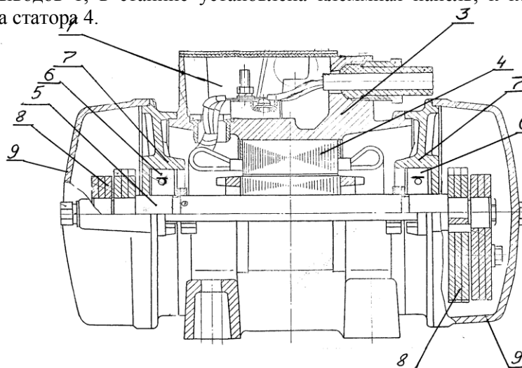
Рис. 2 Устройство вибраторов
