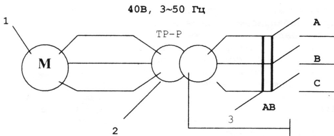
Схема подключения вибратора ВИ-9-8А, ВИ-9-9А
